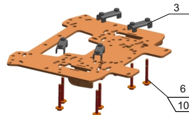
Крепление RM-500, RM-650
