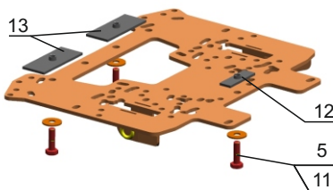
Крепление Polaris Sportsman 570
