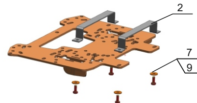
Крепление BRP Outlander G2
